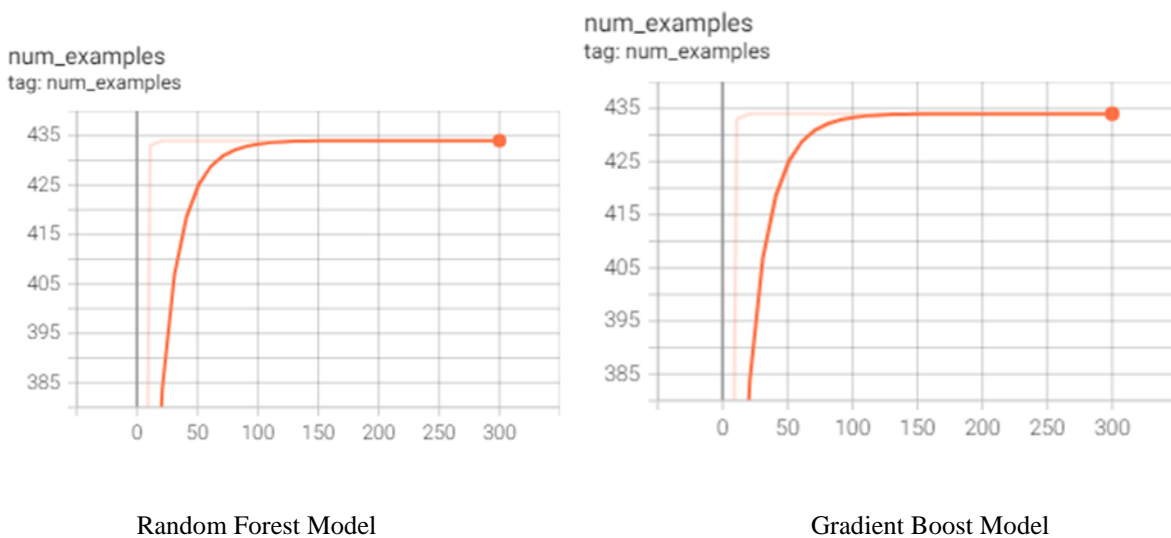
Fig. 15: Num_Examples tag
