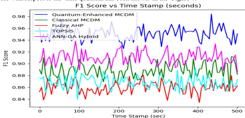
Figure 4. F1 Score versus Time Stamp(sec)
